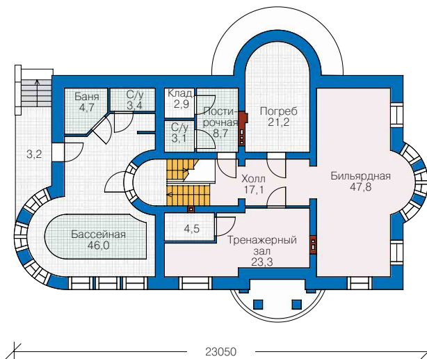
План цокольного этажа
