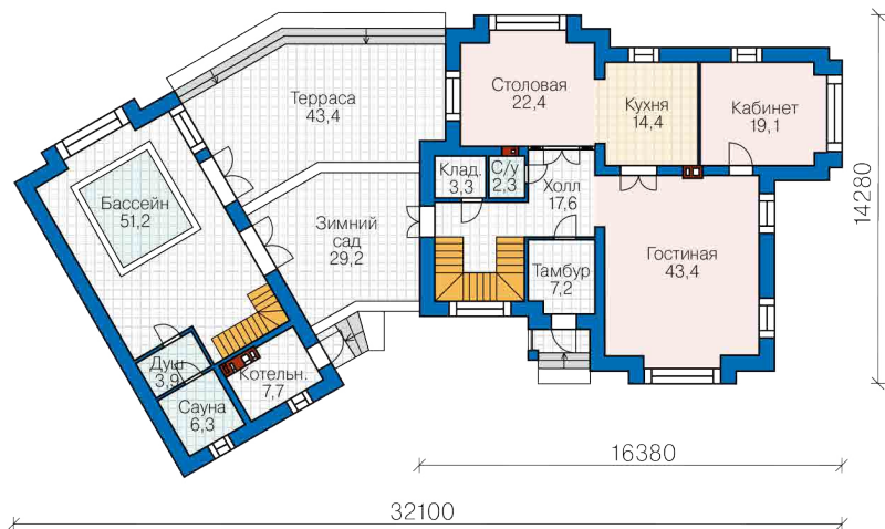
План первого этажа
