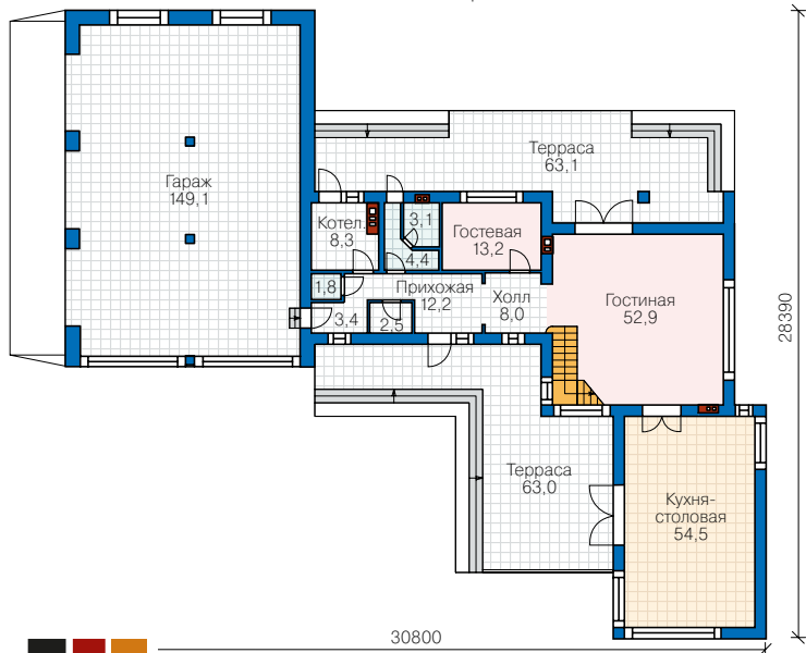
План первого этажа
