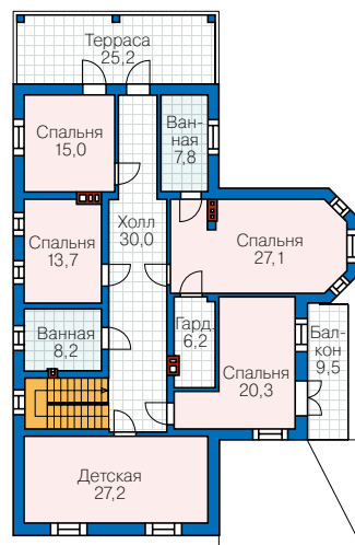
План второго этажа
