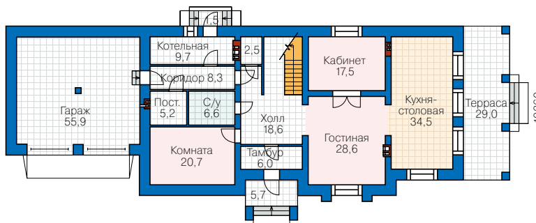
План первого этажа
