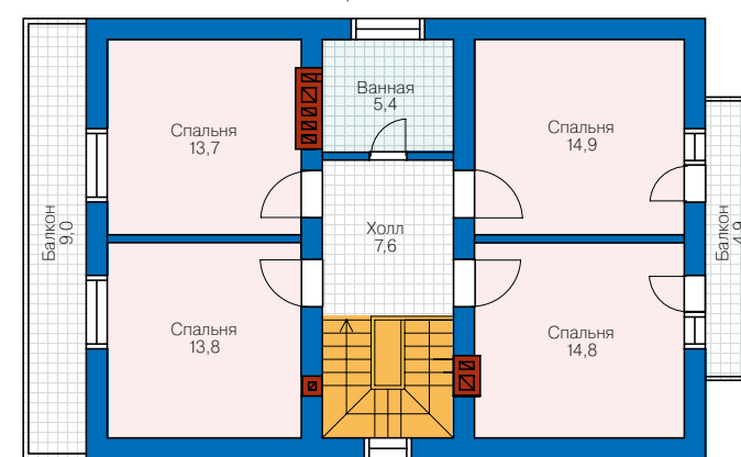
План второго этажа
